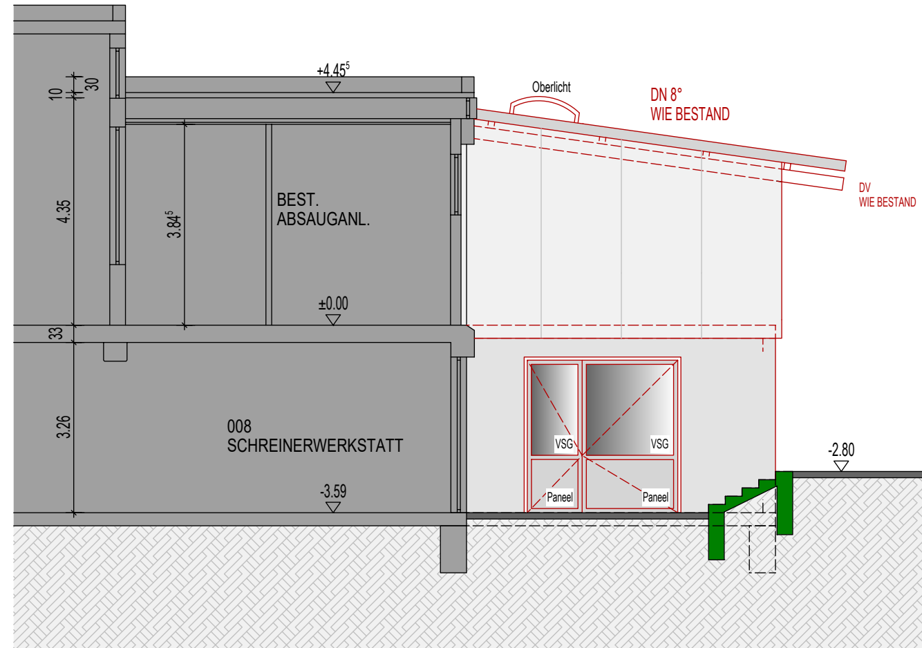
ANSICHT OST
