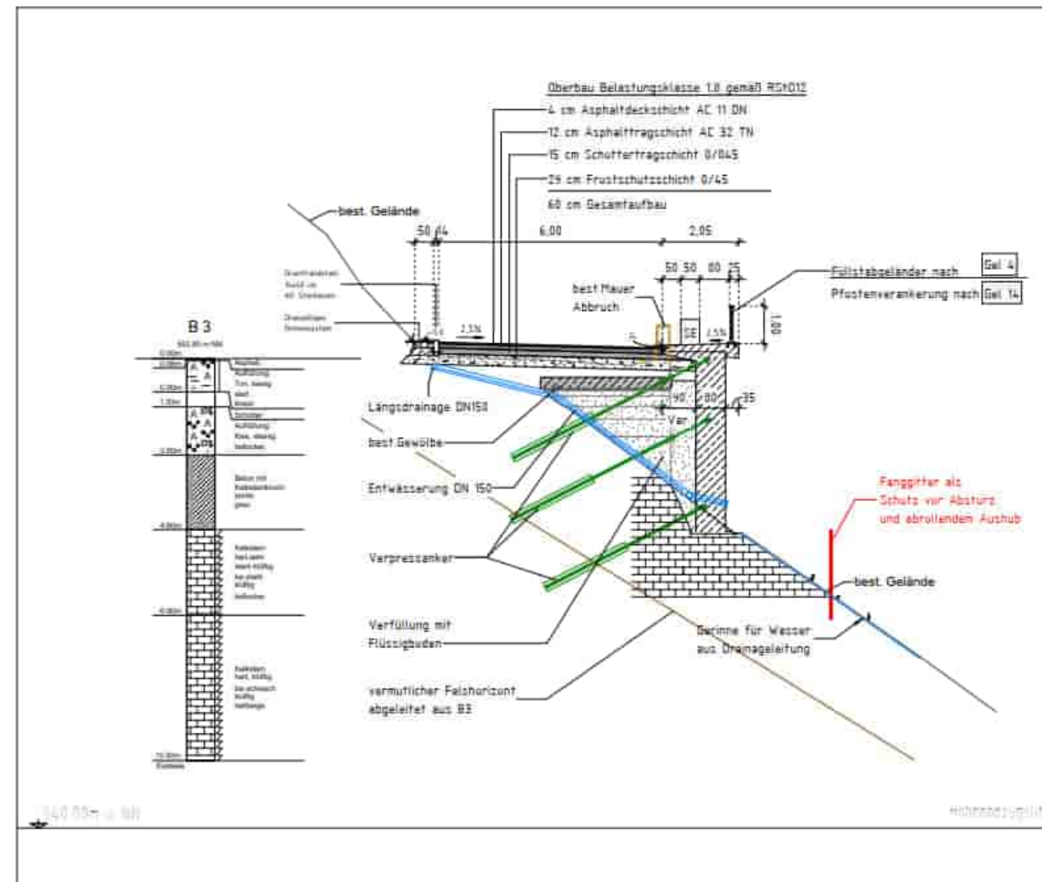
RQ 2 M 1 : 100
