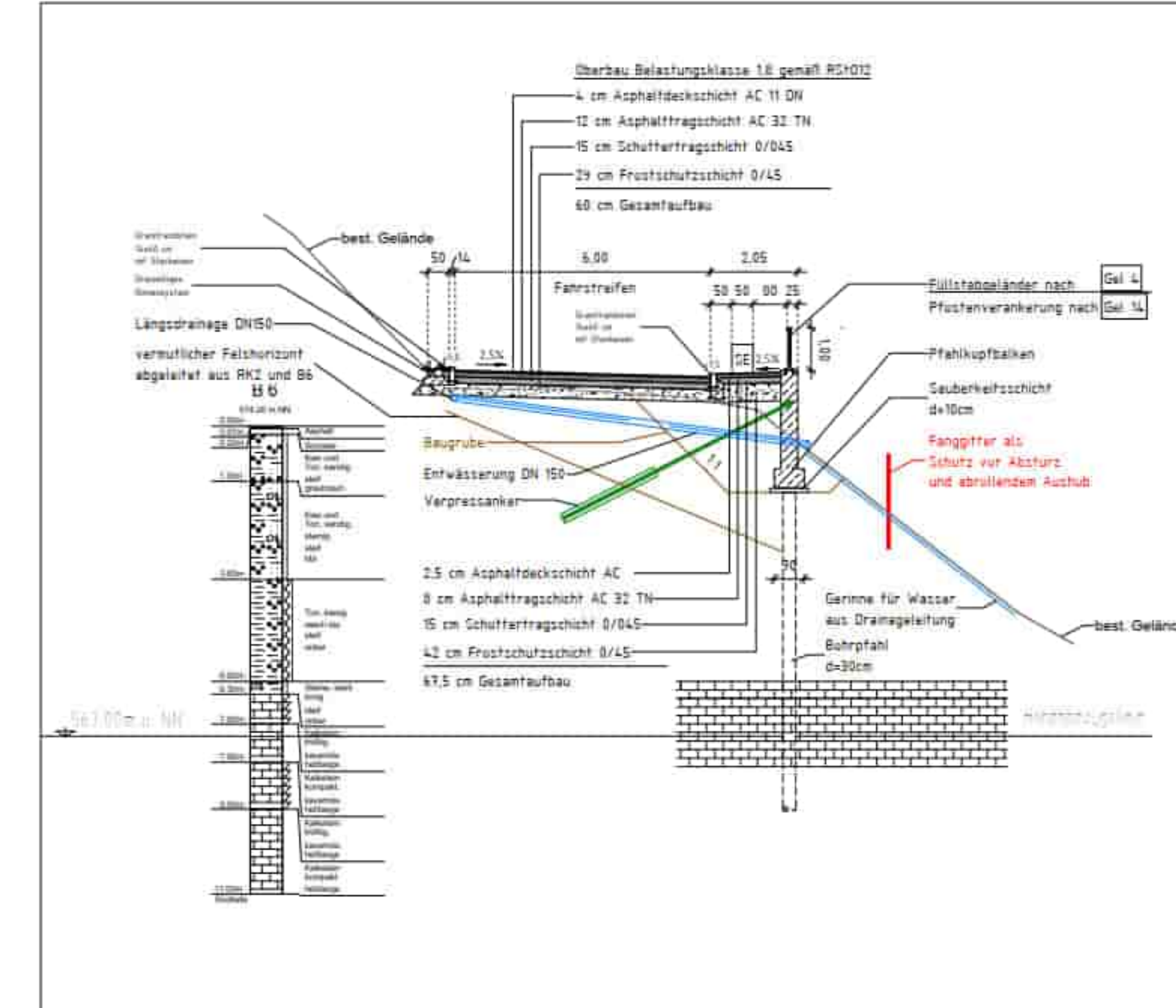
RQ 3 M 1 : 100
